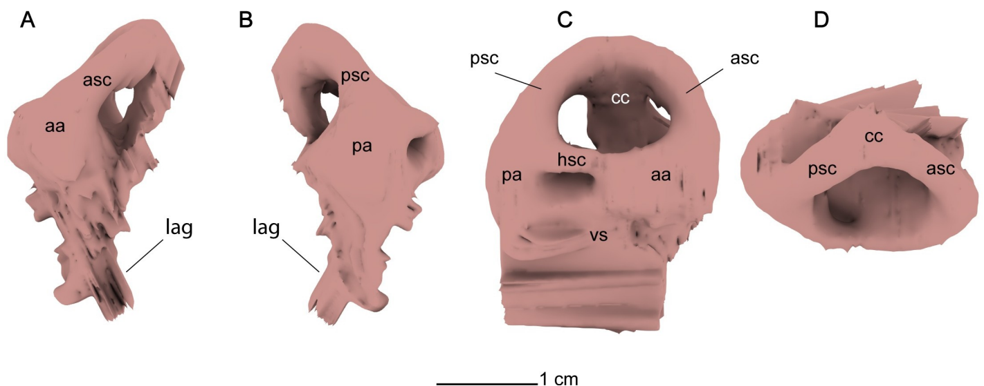
Fig 13. Endosseous labyrinth digital cast of Cardiocrorax mukulu (MGUAN PA278). A. Anterior view. B. Posterior view. C. Ventral view. D. Dorsal view.
